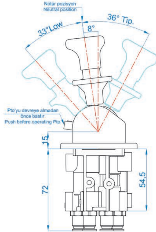
Teknik özellikleri Technical specifications
